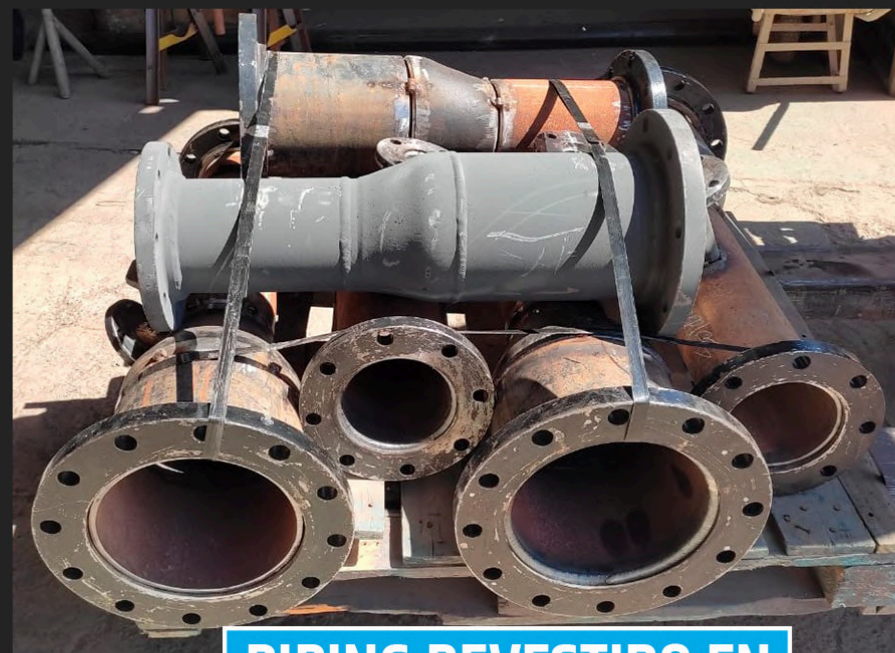
PIPING REVESTIDO EN POLIURETANO
